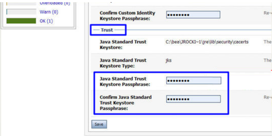
图 4-18 信任库文件
