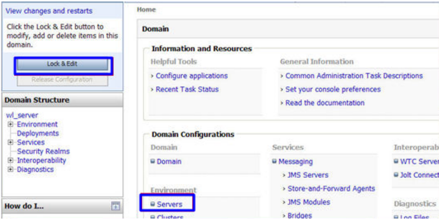
图 4-13 服务器
