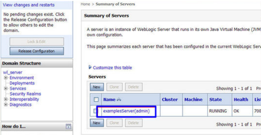
图 4-14 目标服务器
