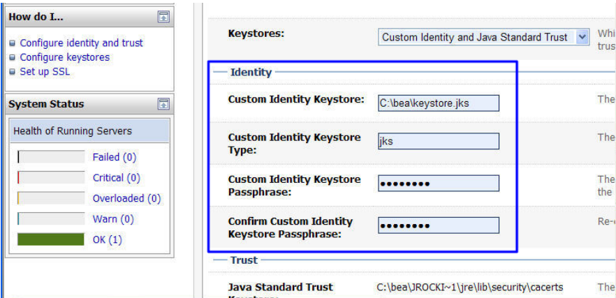
图 4-17 密钥
