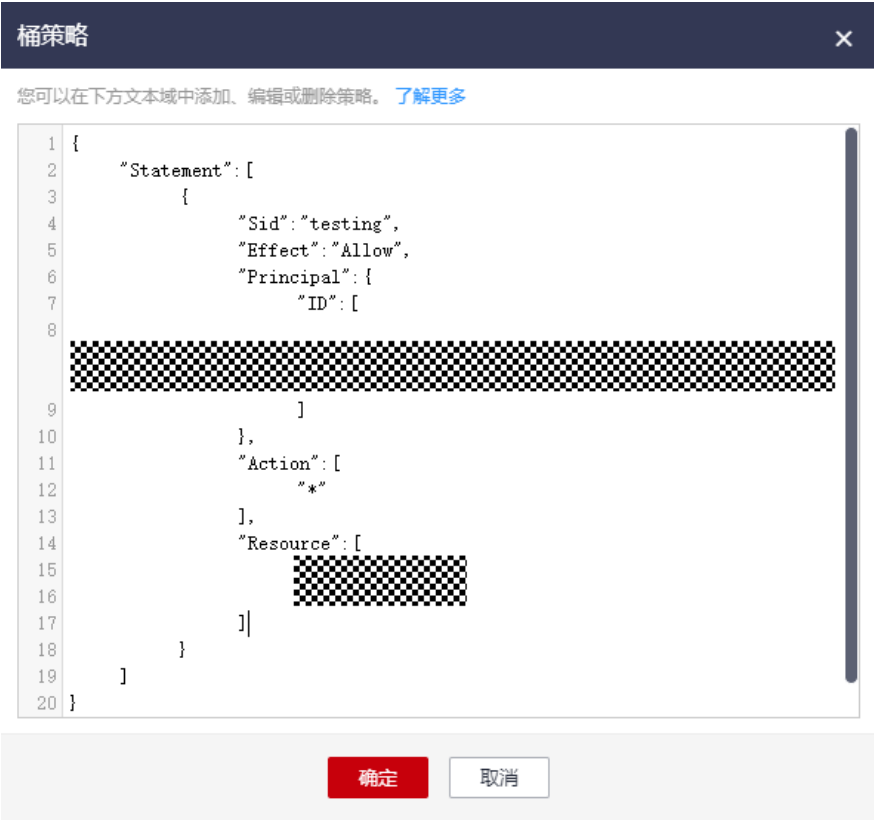
图 7-4 桶策略
